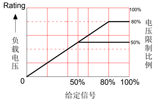
图 7-3b 电压限制
