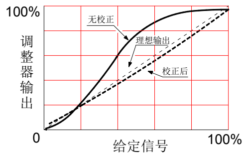
图 7-1 移相
