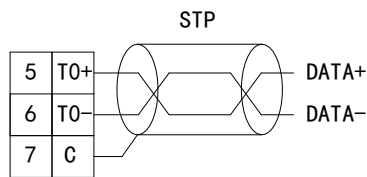
图 3-4 串口接线
