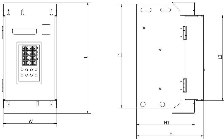
图 3-2 外形尺寸图
